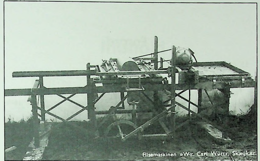
Flisemaskinen "W". Carl Würtz, Skægkær
